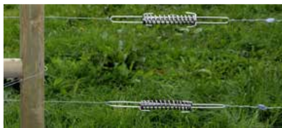
Bilde 14. Spenningsfjær, 90601980.
