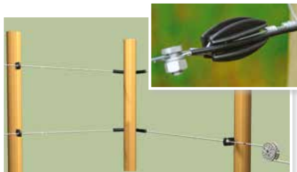
Bilde 5 og 6. Isolatorrør eller eggisolator i hjørnene.
