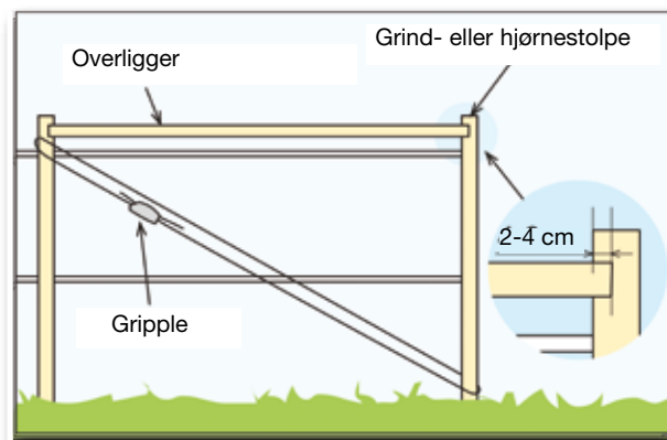
Bilde 3. Alternativ 1 Hjørne-/grindforsterkning med parallellogram. OBS! Det er viktig å lage et 2-4 cm stort uttak i stolpene slik at overliggeren får et sterkt feste.
