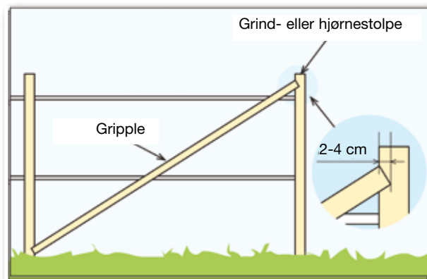
Bilde 4. Alternativ 2 Hjørne-/grindforsterkning med støtte. OBS! Det er viktig å lage et 2-4 cm stort uttak i stolpene slik at festet blir sterkt for støttene.
