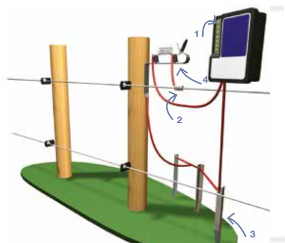
Bilde 25. Monter minst en tordenværbeskyttelse langs gjerdet, så reduseres risikoen for at lyn skader gjerdet.
